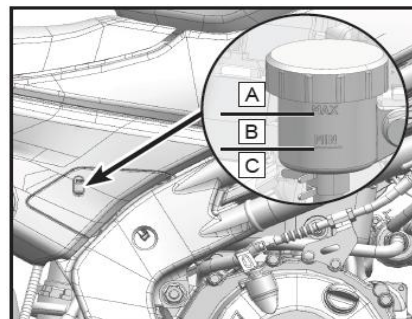
Компенсационный бачок заднего тормозного механизма
